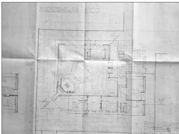
Slika 5.: Tlocrt, prizemlje, Župnog centra Uzvišenja svetog Križa Osijek VI. 41
