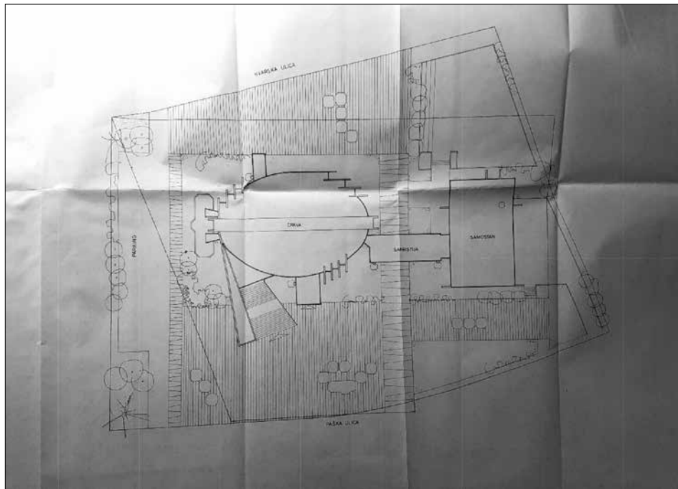
Slika 3.: Situacioni plan u mjerilu 1 : 200 Župni centar sa crkvom Svete Obitelji Jug 2. 35
