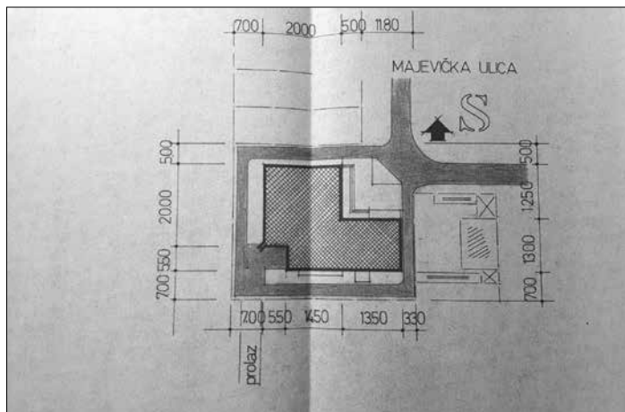
Slika 4.: Situacioni plan Župnog centra Uzvišenja svetog Križa Osijek VI u omjeru 1 : 300. 39
